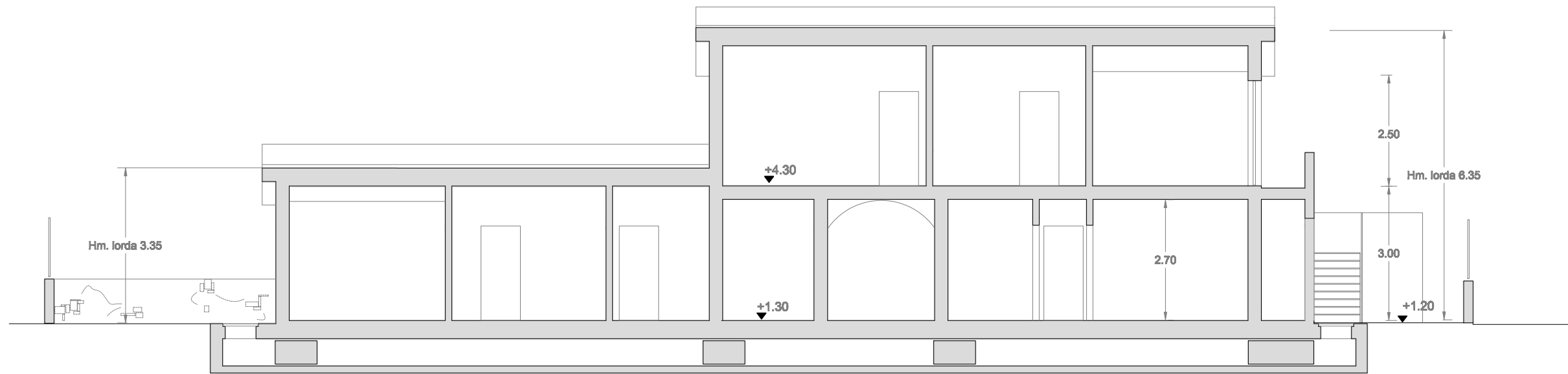
SEZIONE AA 1\100
