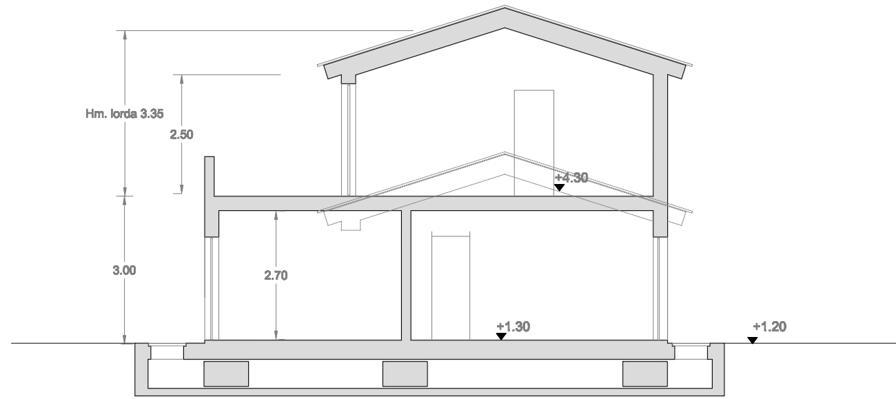
SEZIONE BB 1\100
