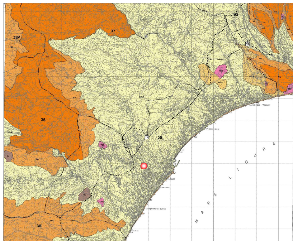
GEOMORFOLOGICO
