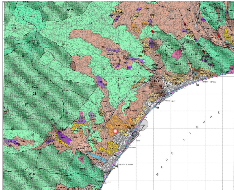
INSEDIATIVO
