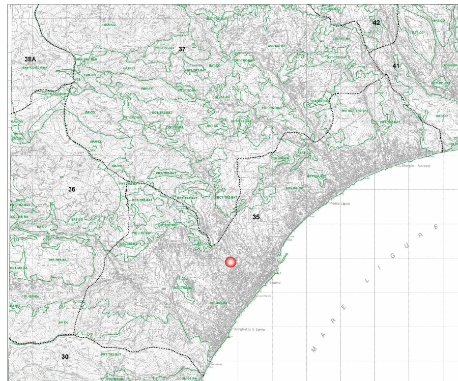
VEGETAZIONALE
